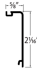
END CAP
