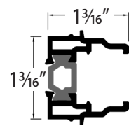
ASTRAGAL
